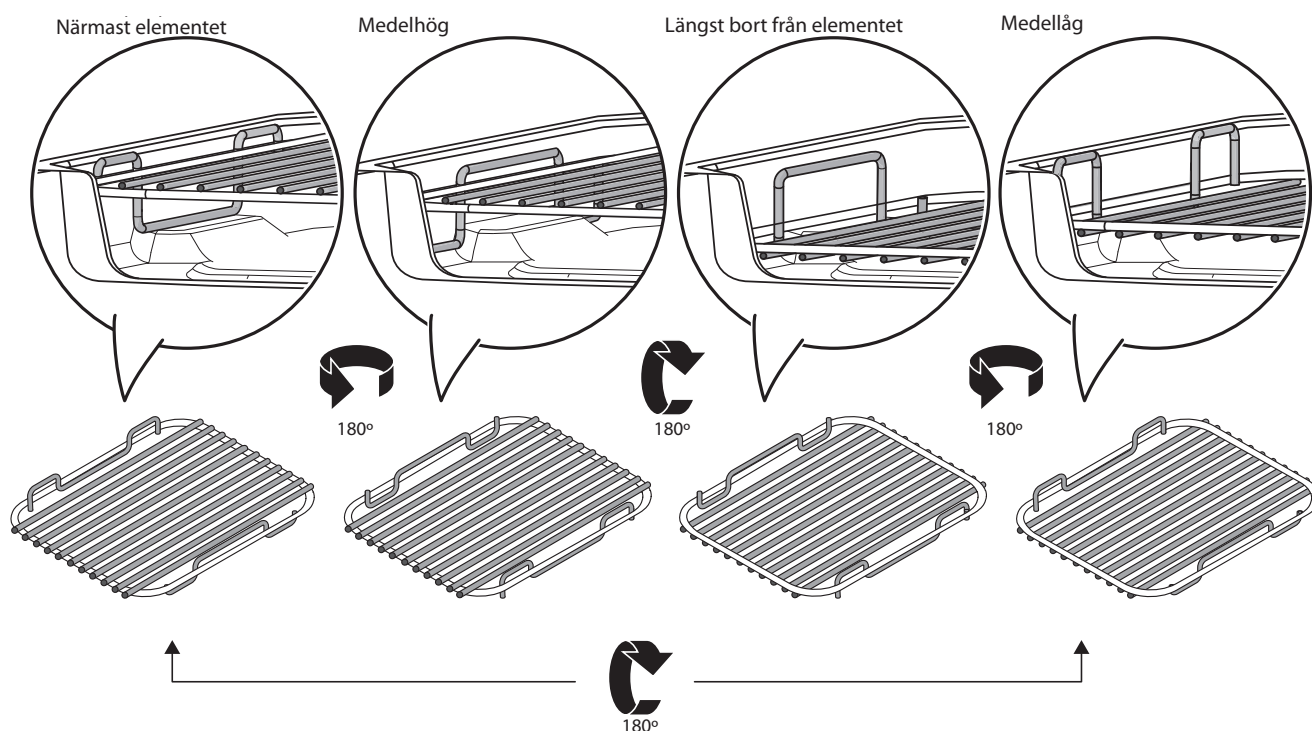
Fyra grillhöjdspositioner
