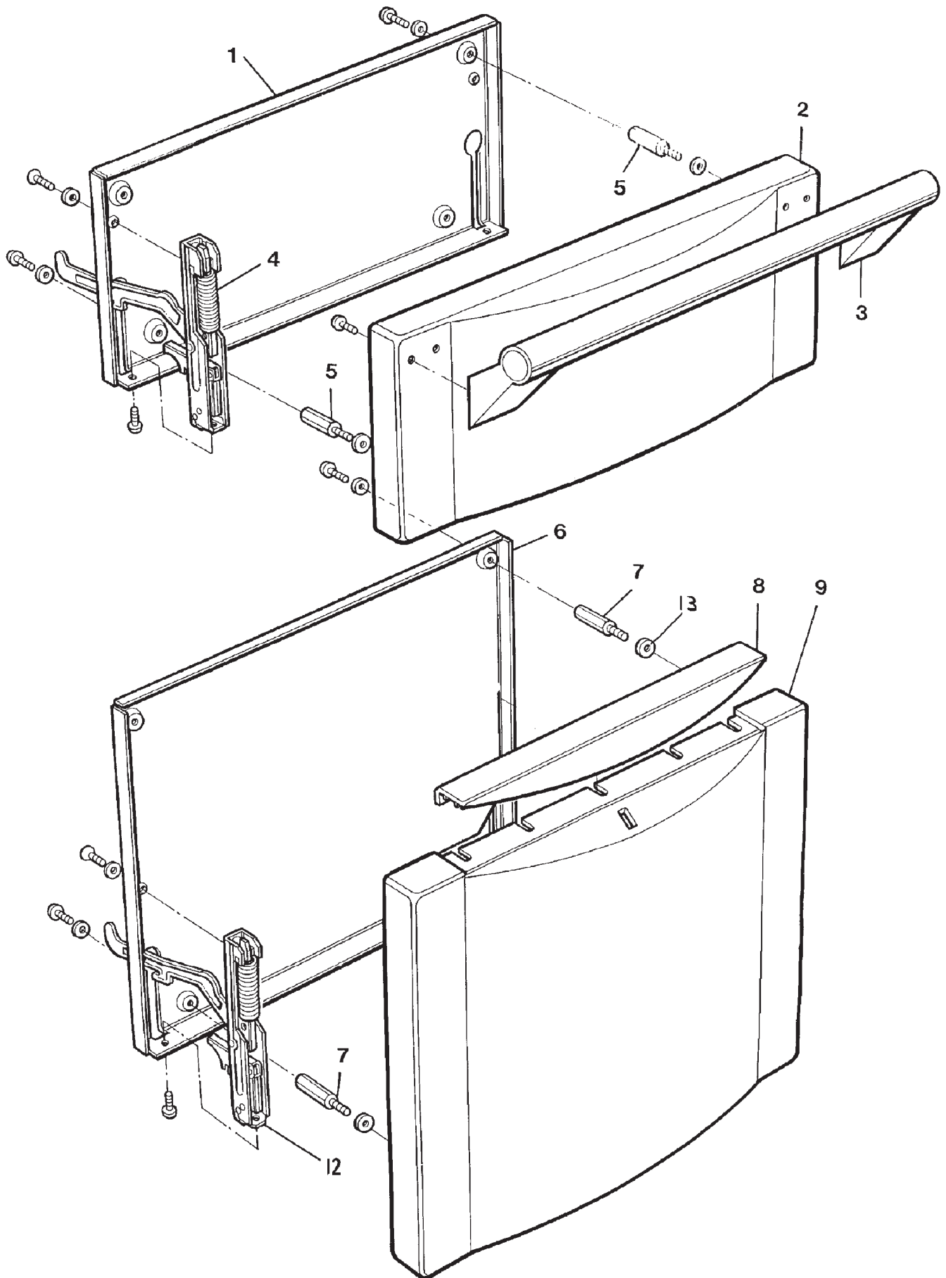
AGA MASTERCHEF - 100DF (FSD) UPPER & LOWER SOLID DOOR ASSEMBLIES
