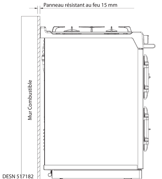
Fig. 12.3 INSTALLATION SUR MUR COMBUSTIBLE À L'AIDE DU PANNEAU RÉSISTANT AU FEU
