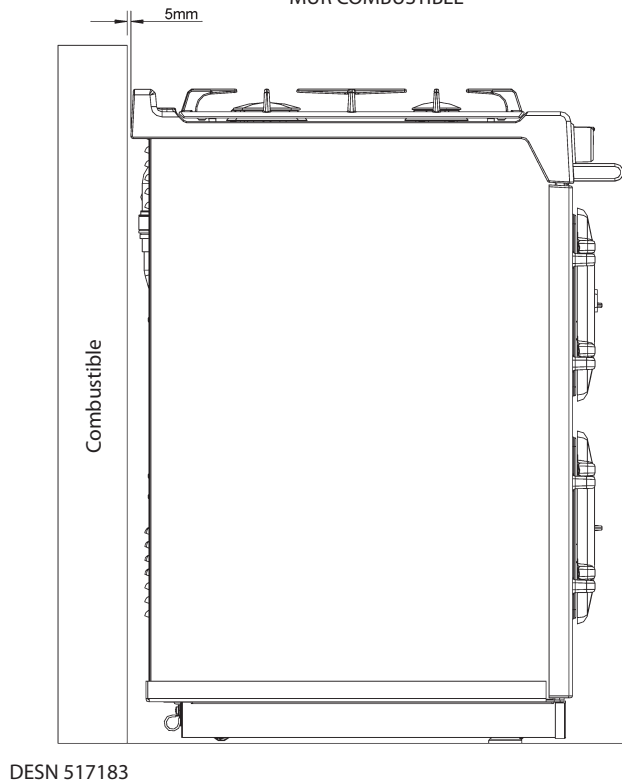
Fig. 12.4 DÉGAGEMENT POUR L'INSTALLATION SUR MUR COMBUSTIBLE
